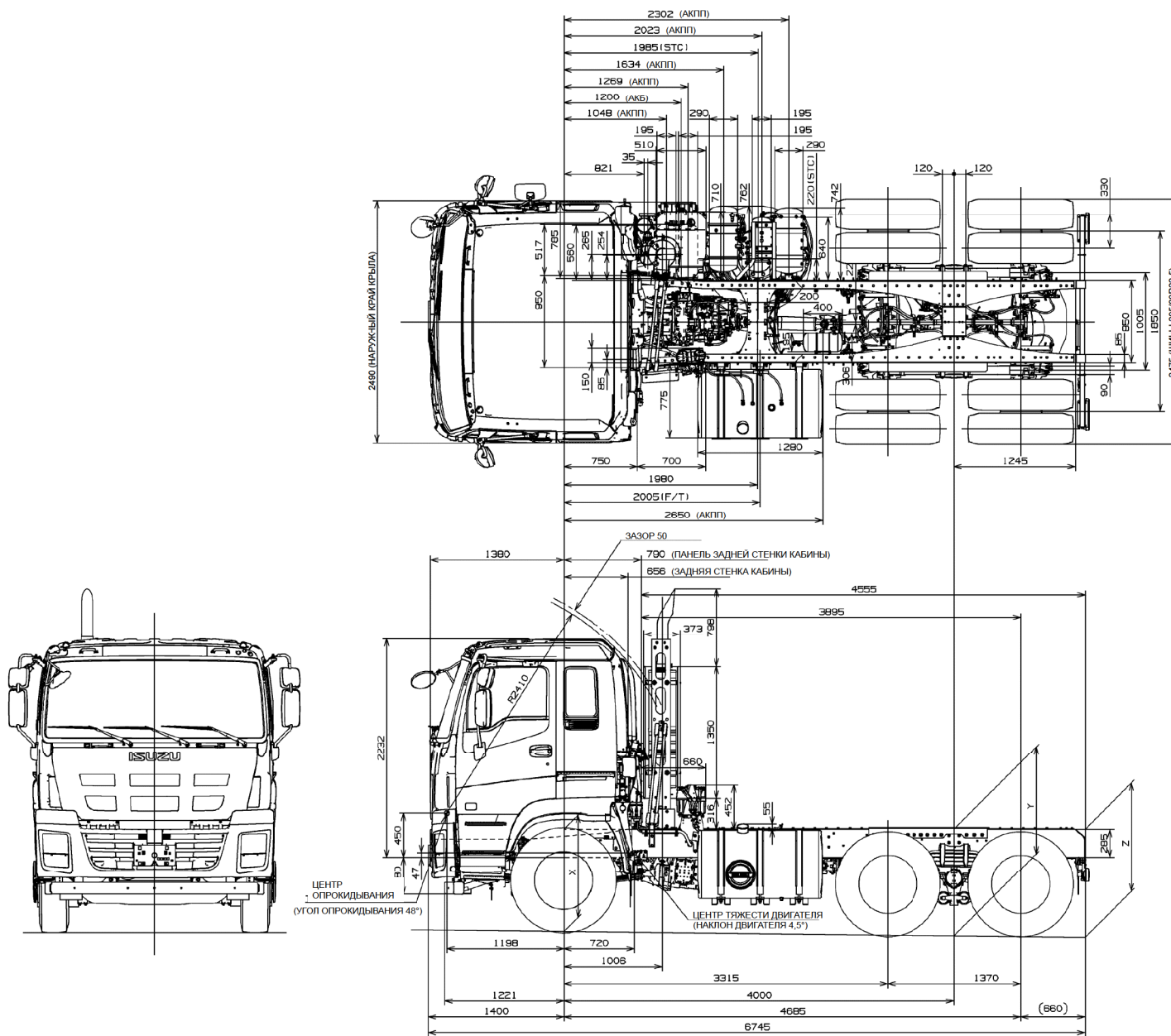
Рис. 9-1-9. Чертеж шасси с кабиной. EXZ52KLX3T17 (выхлопная труба типа «бокс»)
