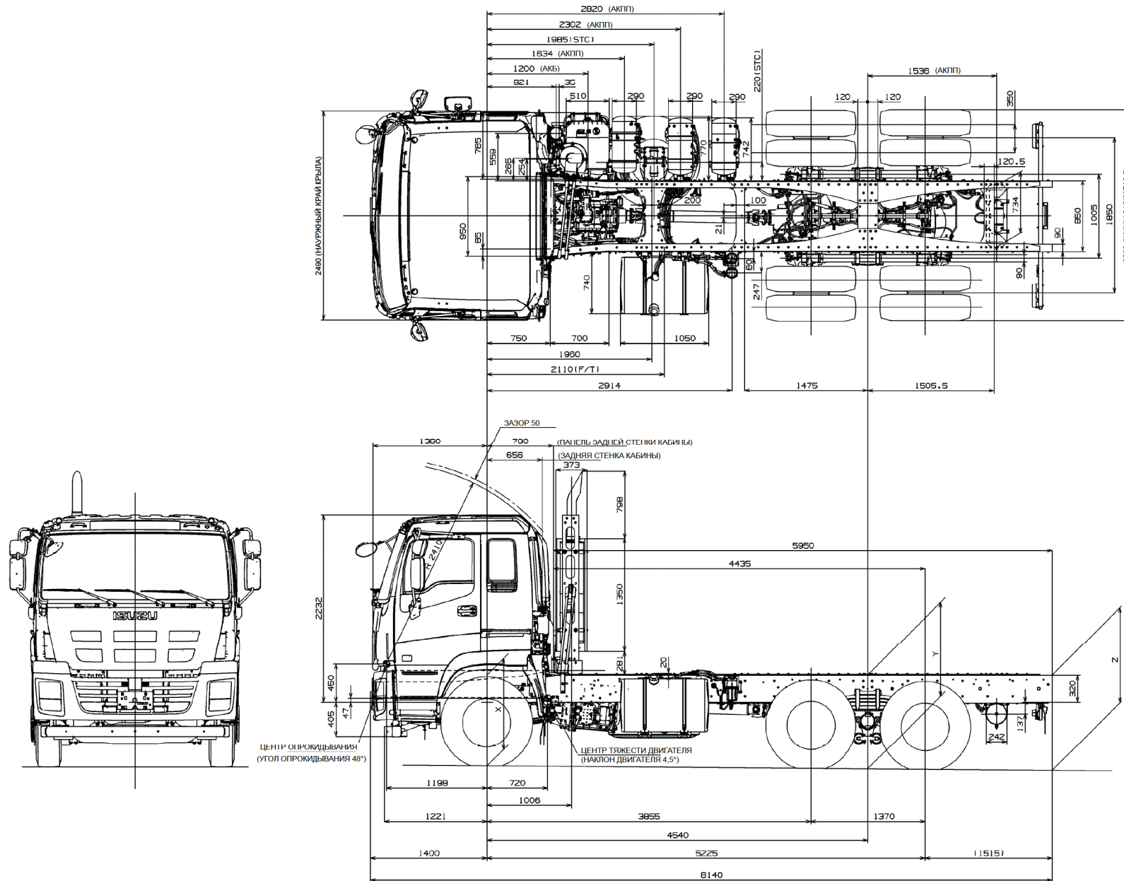
Рис. 9-1-1. Чертеж шасси с кабиной. CYZ52MLD3T17 (КПП типа MJT7S) MJT7S
