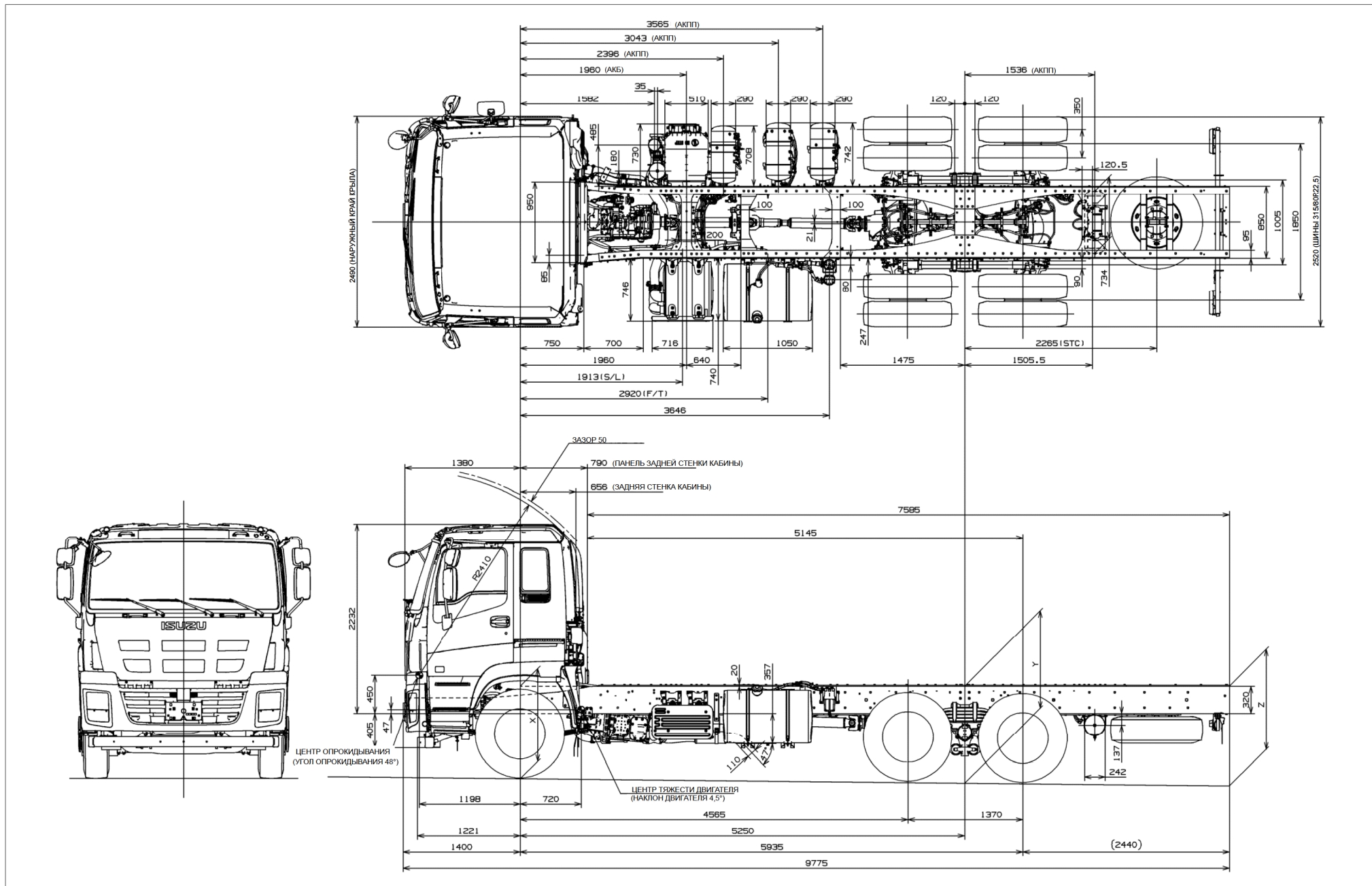
Рис. 9-1-7. Чертеж шасси с кабиной. CYZ52TLC3T17
